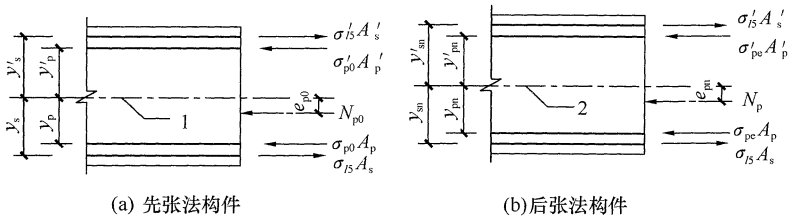
图 5.1.11 预加力作用点位置
