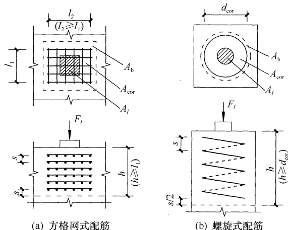
图 5.8.4 局部受压区的间接钢筋
