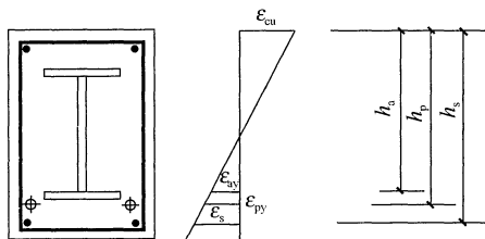
图 8.2.2 界限受压区高度计算简图
