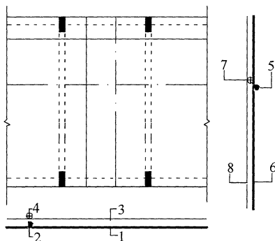
图 11.1.4 预应力筋与普通钢筋的位置关系
