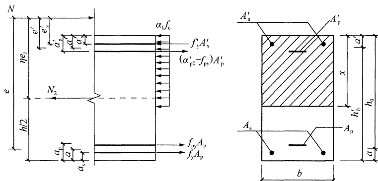
图 5 矩形截面偏心受压构件正截面受压承载力计算
