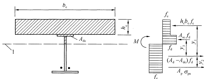
图 8.2.6-2 塑性中和轴在钢梁内时的组合梁截面及应力图形
