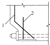
图 5.8.1 端部凹进处 构造配筋
