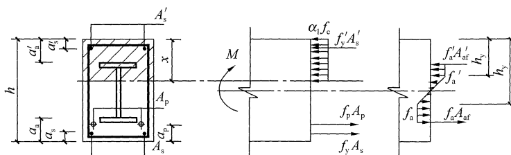
图 8.2.3 框架梁正截面受弯承载力计算
