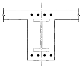
图 8.1.1 预应力型钢混凝土梁的截面配筋形式
