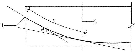
图 4.3.6 预应力摩擦损失计算 1—张拉端；2—计算截面
