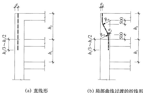
图 11.1.2 柱预应力筋束形
