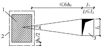
图 5.7.2 邻近孔洞时的计算截面周长
