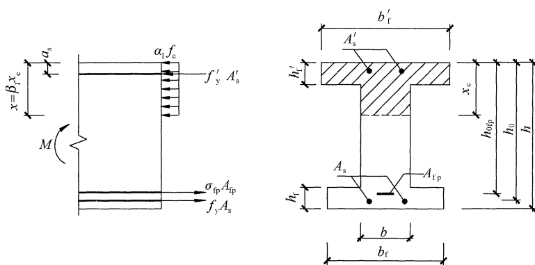
图 10.3.4-2 受弯构件正截面受弯承载力计算
