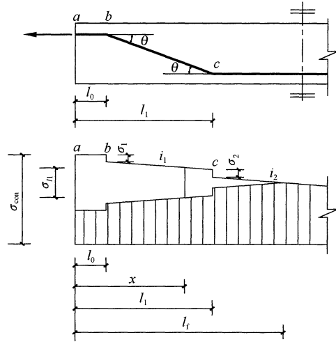
图 4.3.5-3 折线形预应力筋的预应力损失 \sigma_{11}
