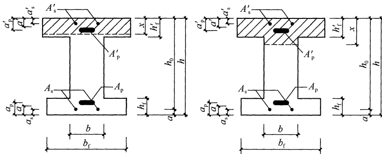
图 3 矩形截面受弯构件正截面受弯承载力计算
