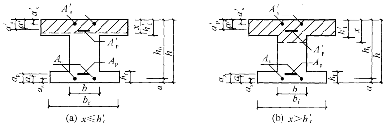
图 5.2.2 T形、I形截面受弯构件受压区高度位置
