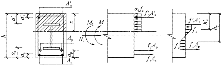
图 8 预应力型钢混凝土构件正截面受弯承载力计算
