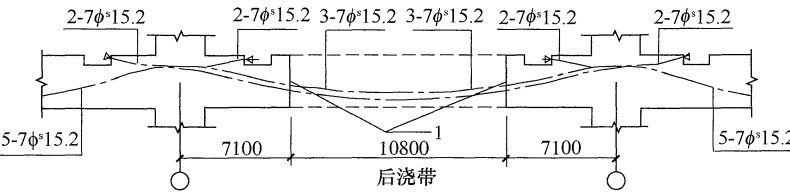
1-锚具连接器
