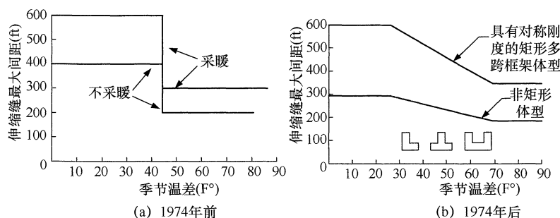
图 6 建筑结构最大不设缝长度
