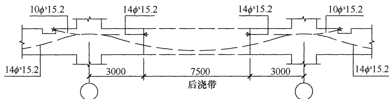
(c) 预应力筋分离连接
