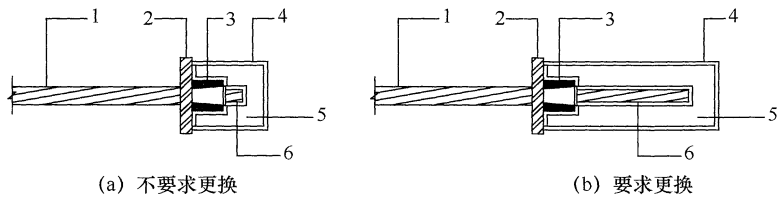
图 9.4.11 锚具防护罩
