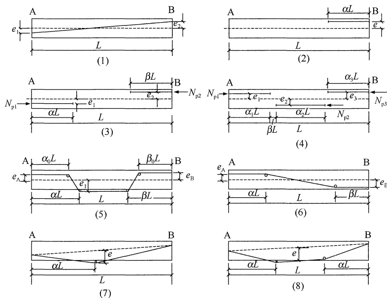
图 B.0.1 体外预应力筋线型布置图
