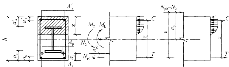
图 8.3.2 预应力型钢混凝土框架梁最大裂缝宽度计算简图
