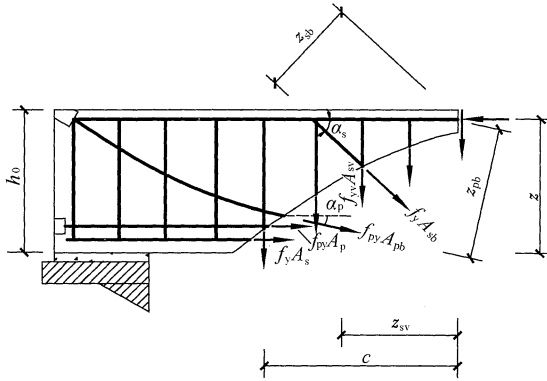
图 5.5.8 受弯构件斜截面受弯承载力计算
