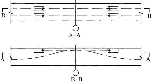
(b) 预应力筋交叉搭接
