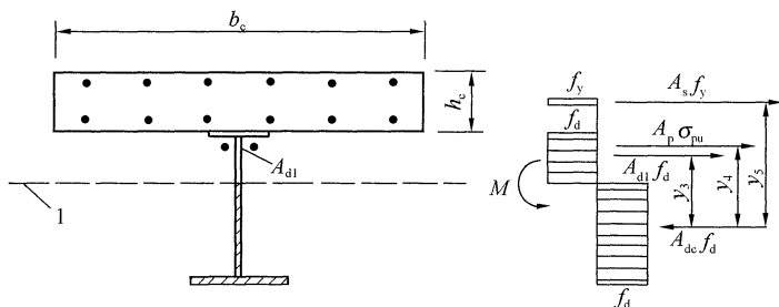
图 8.2.6-3 负弯矩作用时的组合梁截面及应力图形
