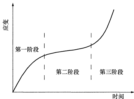
图 1 纤维增强复合材料筋徐变变形的三个阶段
