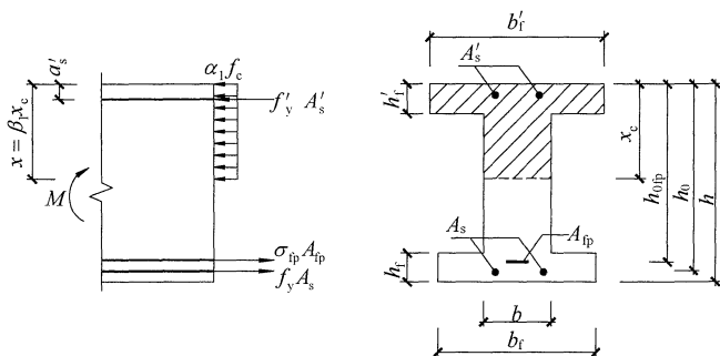
图 10.3.4-1 受弯构件正截面受弯承载力计算
