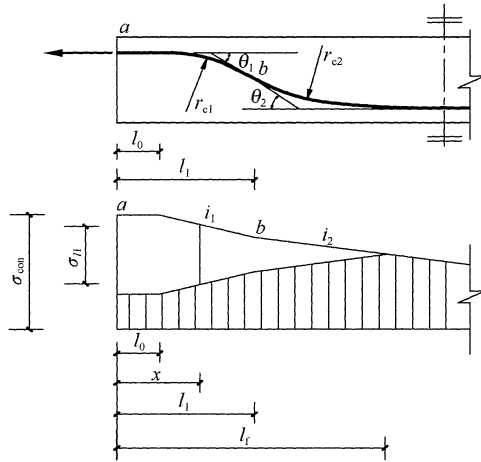
图 4.3.5-2 两条圆弧形曲线组成的预应力筋的预应力损失 \sigma_n
