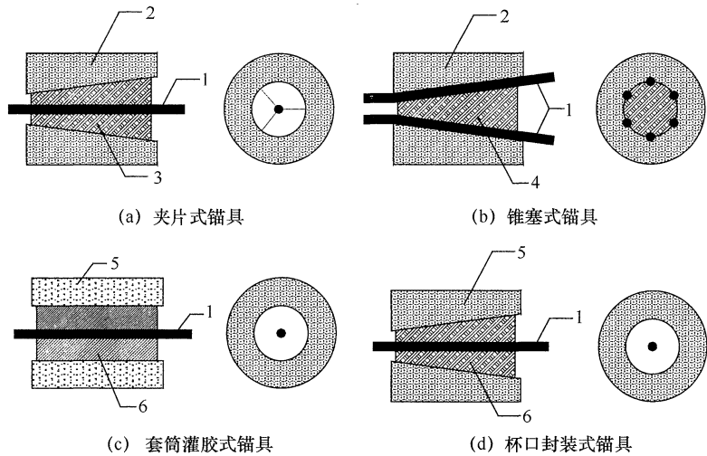
图 2 纤维增强复合材料预应力筋锚具
