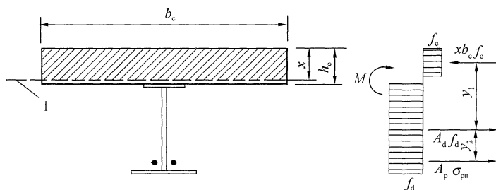
图 8.2.6-1 塑性中和轴在混凝土板内时的组合梁截面及应力图形
