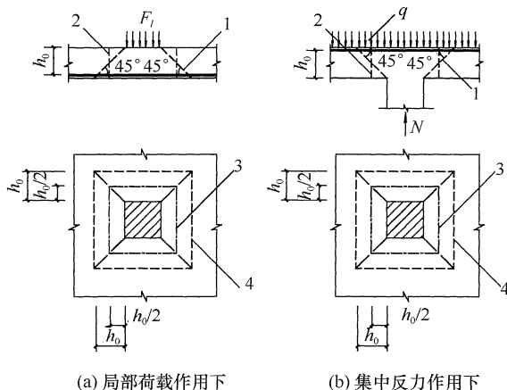
图 5.7.1 板受冲切承载力计算
