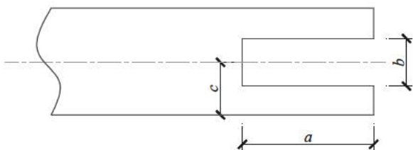
图 9.2.2-2 豁口示意图
