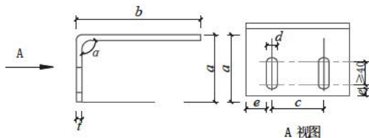
图 9.3.3 连接件、支承件尺寸示意图
