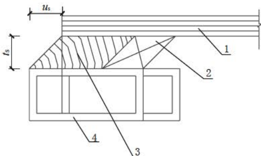
图 5.6.5 硅酮结构密封胶粘接厚度示意
