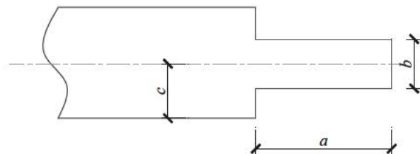
图 9.2.2-3 榫头示意图
