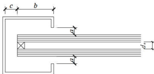
图 9.5.3 中空玻璃与槽口的配合示意
