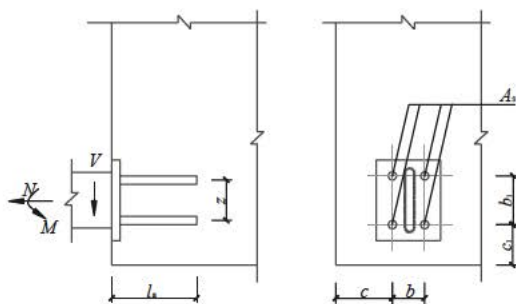
图 C 锚板和直锚筋组成的预埋件
