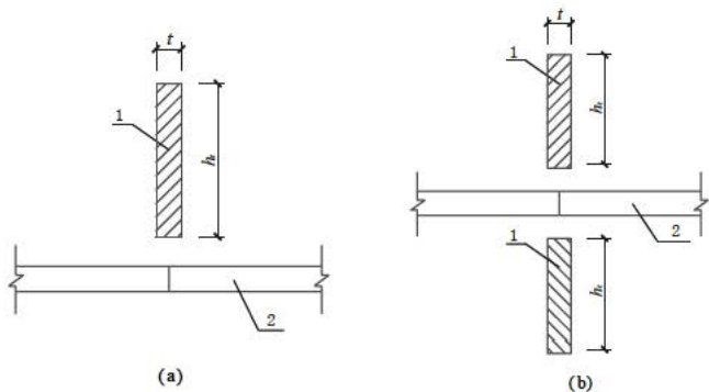
图 7.3.2 全玻璃幕墙玻璃肋截面尺寸示意
