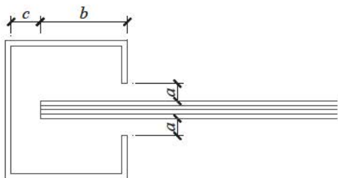
图 9.5.2 单层玻璃与槽口的配合示意
