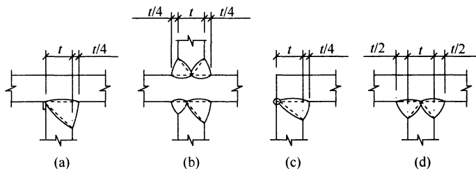
图 6.4.1 焊脚尺寸
