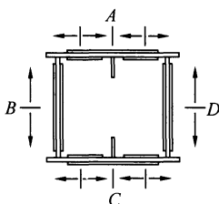
图 2 箱形节点施拧顺序
