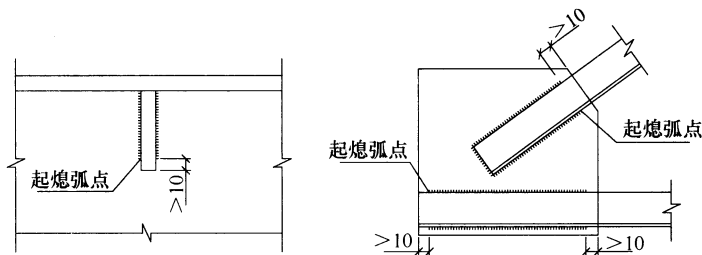
图 6.4.6 起熄弧点位置
