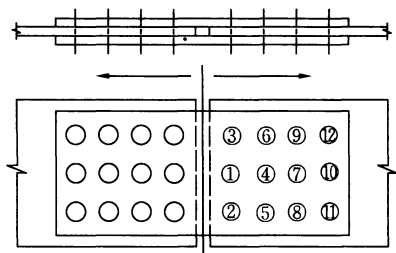
图 1 一般节点施拧顺序
