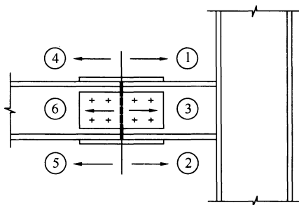
图 3 工字梁节点施拧顺序
