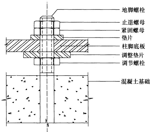
图4 柱脚底板标高精确调整
