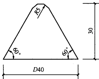
图 13.2.2 加荷头端部尺寸示意
