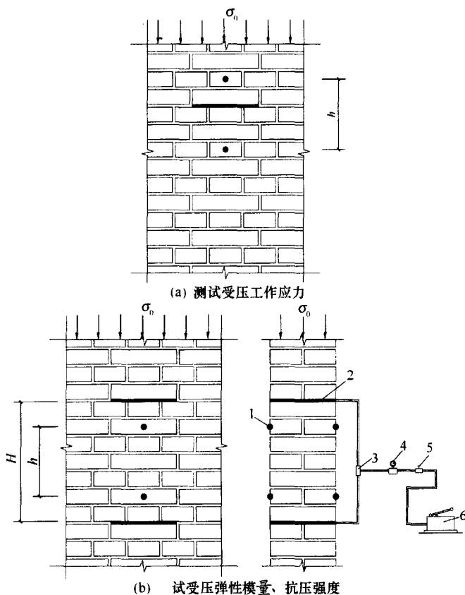
图 5.1.1 测扁顶法测试装置与变形测点布置
