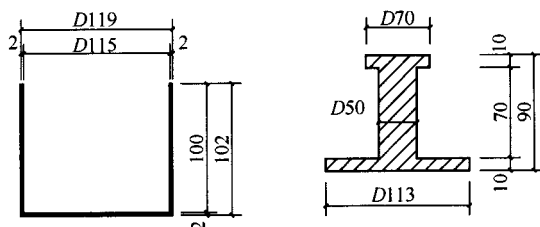
(a) 承压筒剖面
