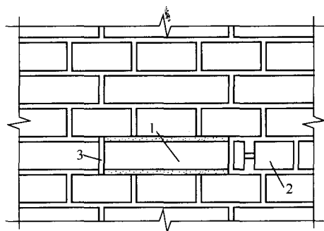
图 8.1.1 原位双剪法测试示意
