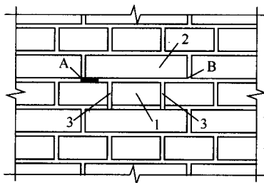
图 9.3.1 试件加工步骤示意
