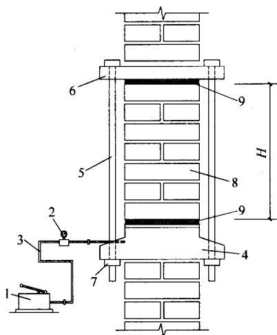
图 4.1.1 原位轴压法测试装置
