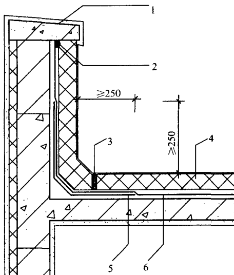
图 5.3.3-1 低女儿墙、山墙防水保温构造
