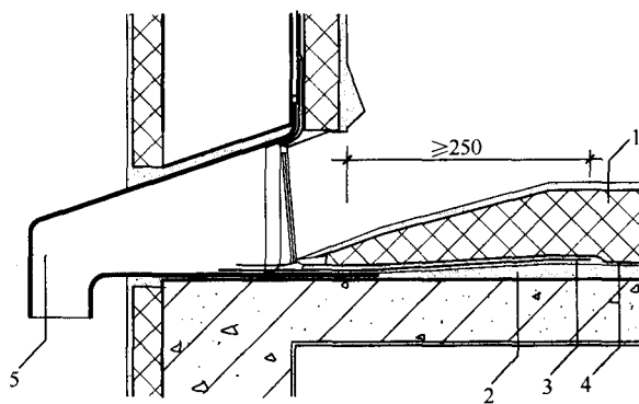
图 5.3.6-2 侧水落口处防水保温构造
