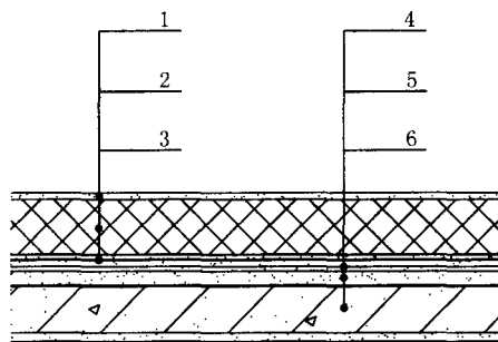
图 5.1.2 倒置式屋面基本构造
