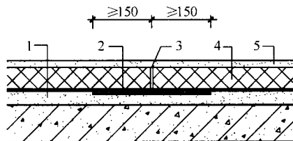
图 5.3.12 聚氨酯防水保温复合板板缝构造
