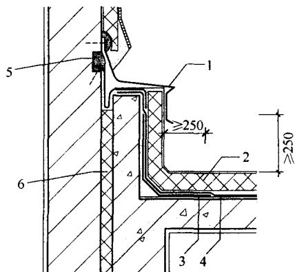
图 5.3.5 屋面高低跨变形缝处防水保温构造
