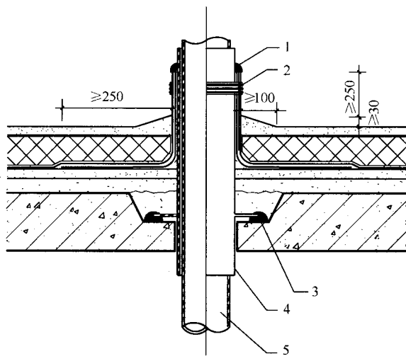
图 5.3.8 伸出屋面管道防水保温构造
