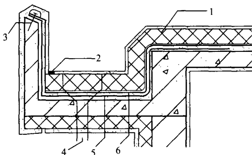
图 5.3.2 天沟、檐沟的防水保温构造
