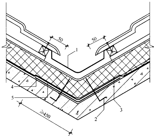
图 5.3.11 瓦屋面天沟防水保温构造
