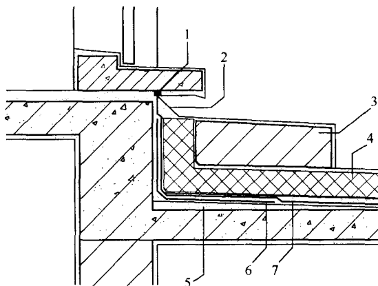
图 5.3.7-1 屋面水平出入口处防水保温构造
