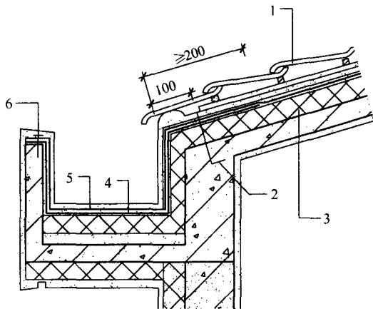
图 5.3.10 瓦屋面檐沟防水保温构造
