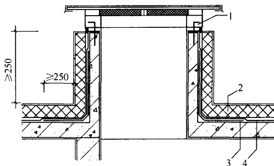
图 5.3.7-2 屋面垂直出入口处防水保温构造
