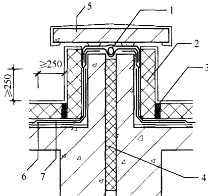
图 5.3.4 屋面变形缝处防水保温构造
