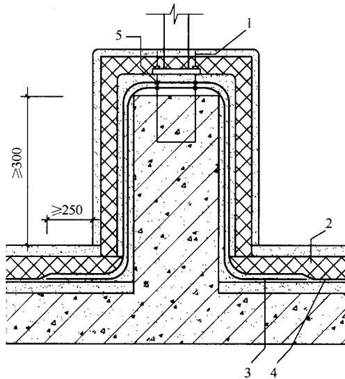
图 5.3.9 屋面设施基座的防水保温构造
