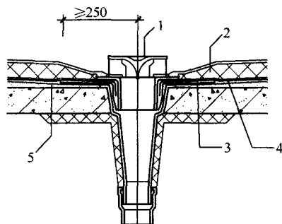
图 5.3.6-1 直排水落口处防水保温构造
