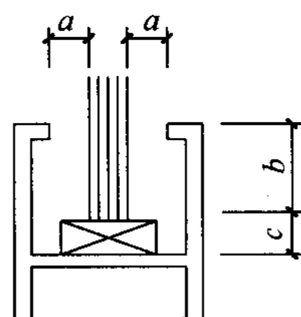
图 5.3.2-1 单片玻璃、夹层玻璃、真空玻璃最小安装尺寸 a —前、后余隙； b —嵌入深度； c —边缘余隙
