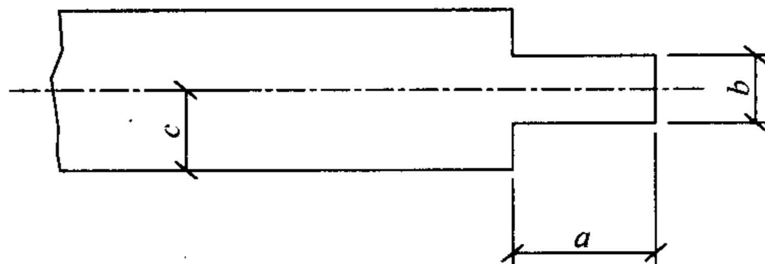
图 6.2.2-2 构件的豁口加工
