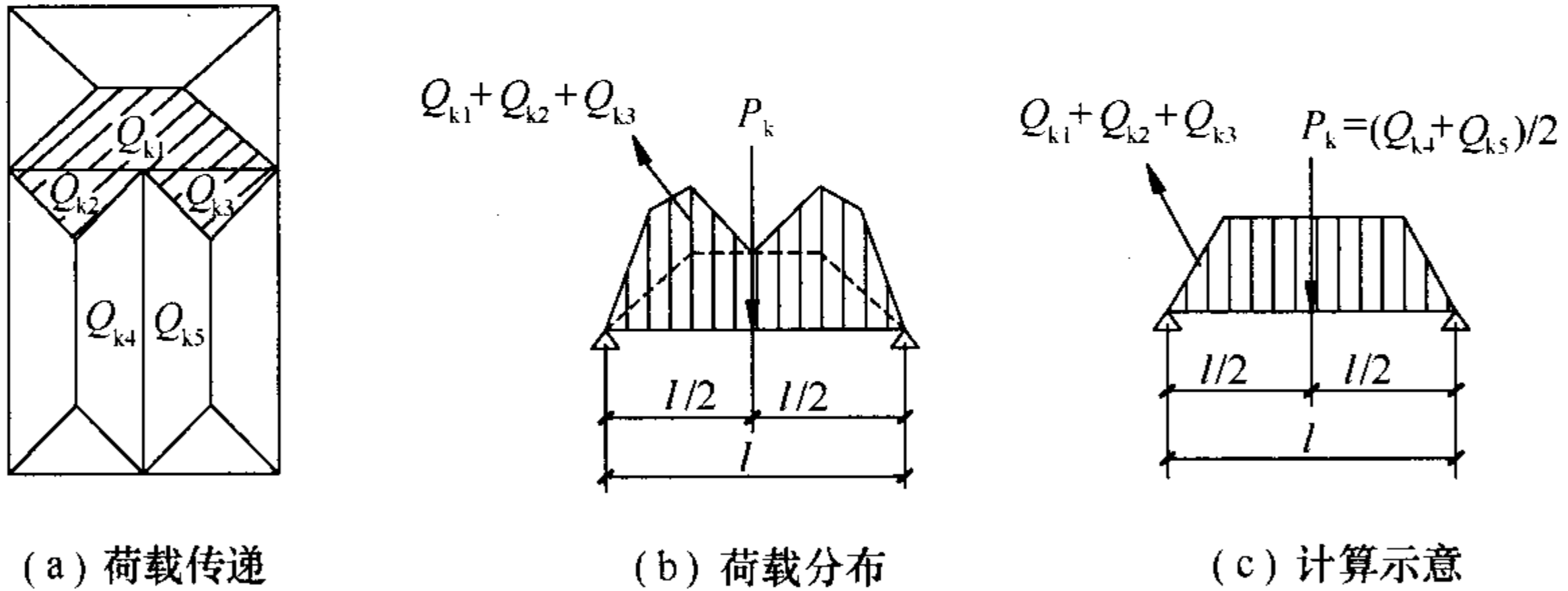
图 B.0.1-4 带上亮双扇门窗荷载传递
