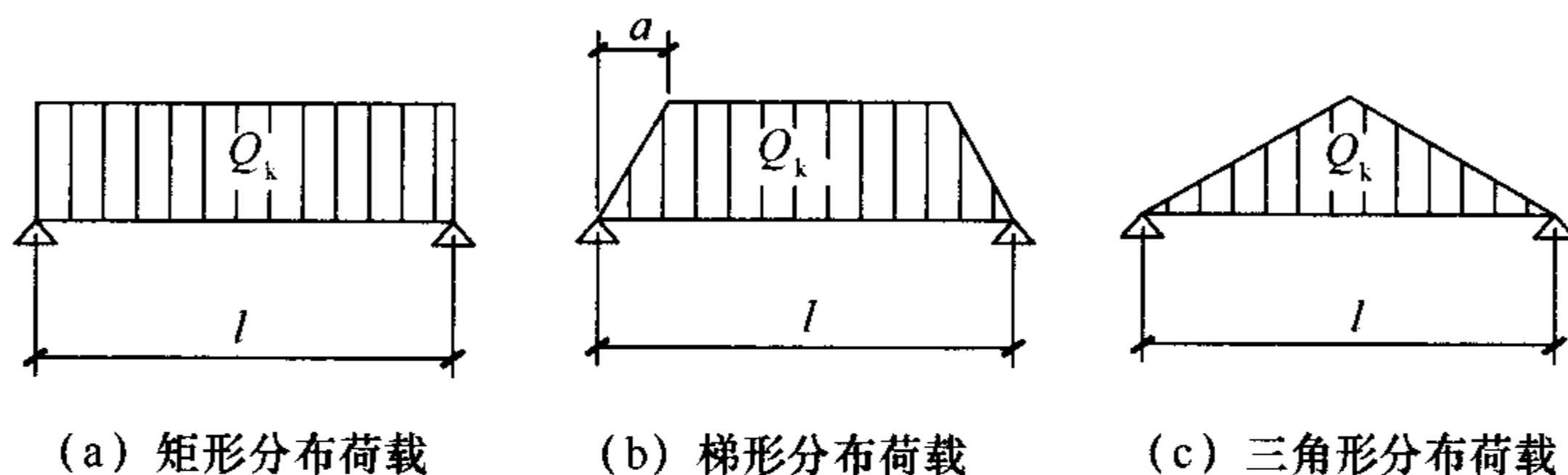
图 B. 0. 2-1 荷载分布
