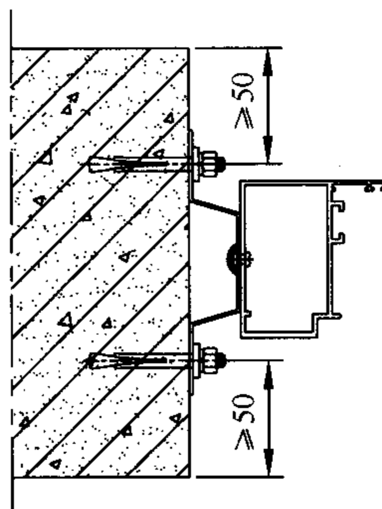
图 7.3.2-2 自攻螺钉连接方式
