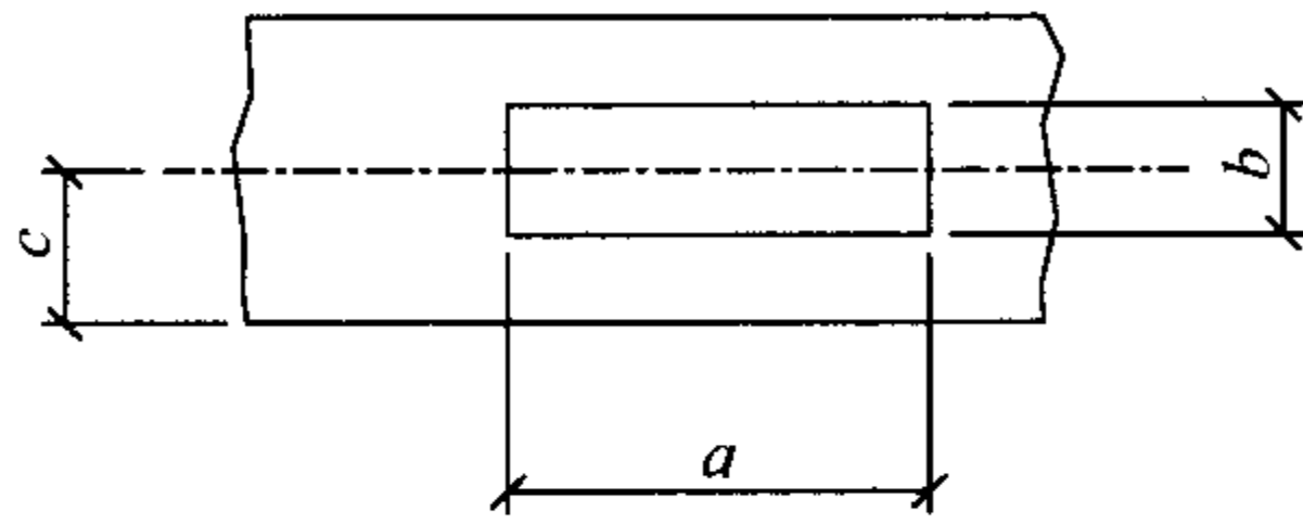
图 6.2.2-1 构件的槽口加工
