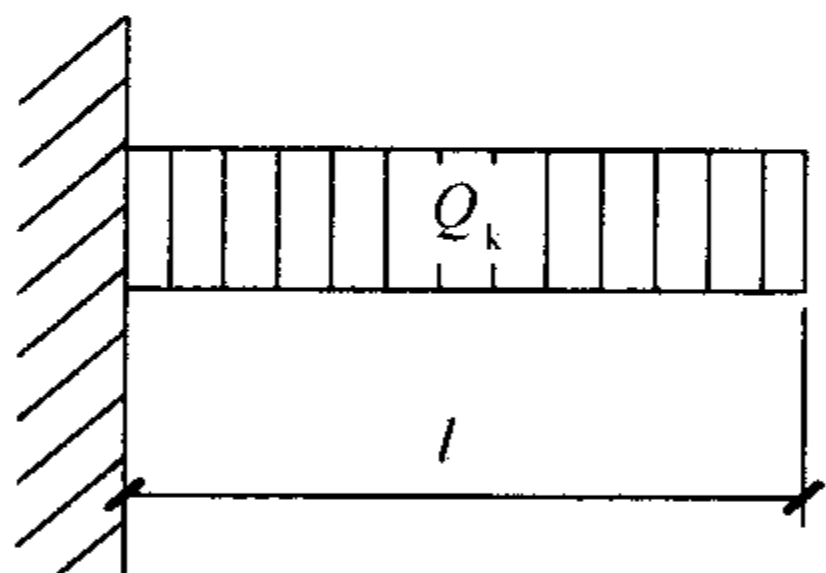
图 B. 0. 1-6 悬臂梁 矩形分布荷载
