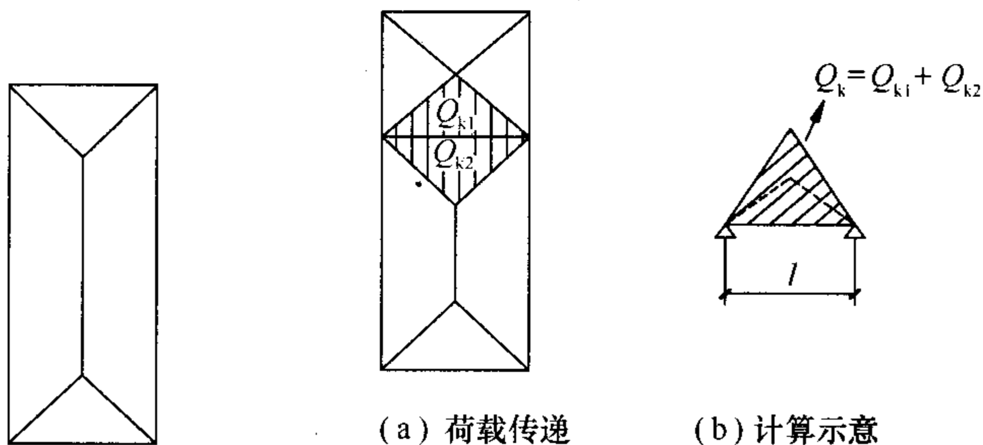
图 B.0.1-1 单扇门窗荷载传递
