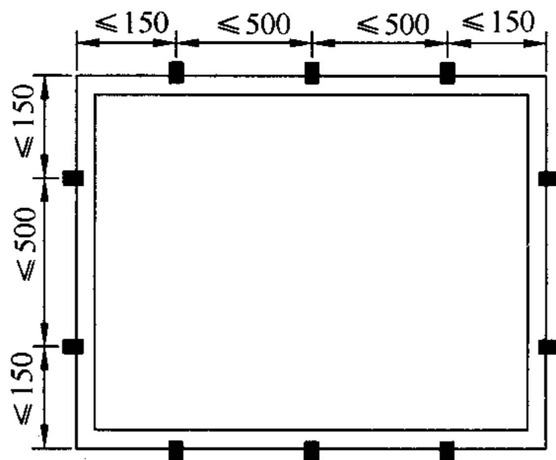
图 7.3.1-1 固定片安装位置
