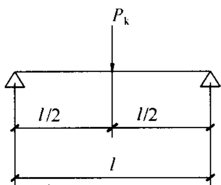
(a) 集中荷载作用于跨中
