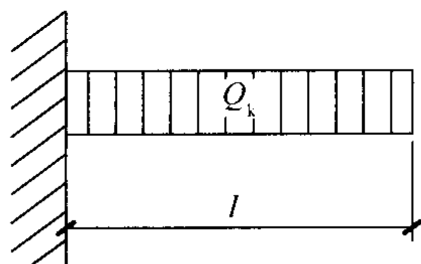
图 B. 0. 2-2 荷载分布
