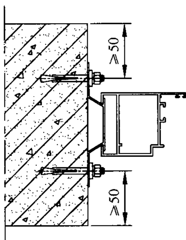
图 7.3.2-1 卡槽连接方式
