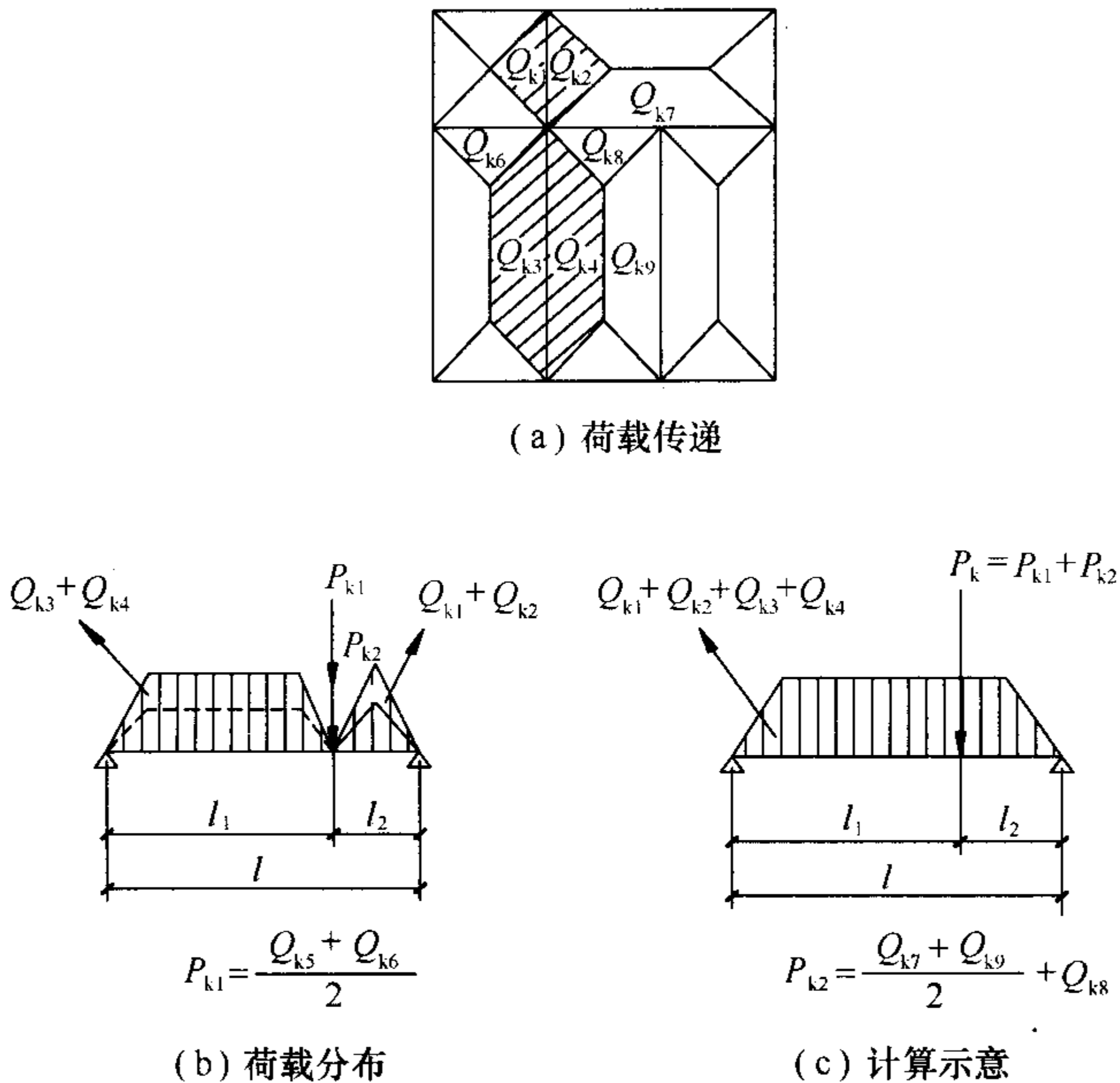
图 B.0.1-5 带上亮多扇门窗荷载传递
