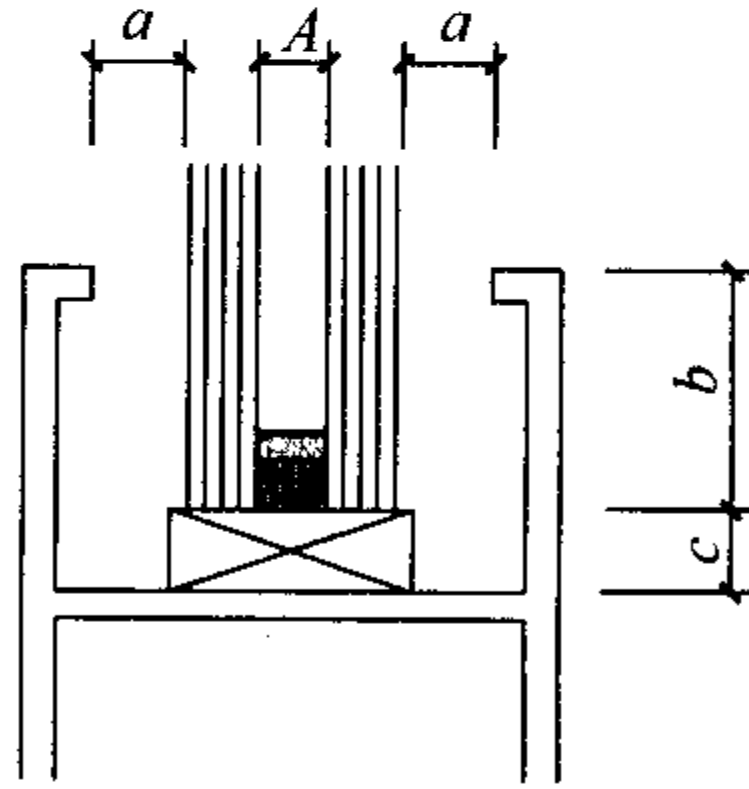
图 5.3.2-2 中空玻璃最小安装尺寸
