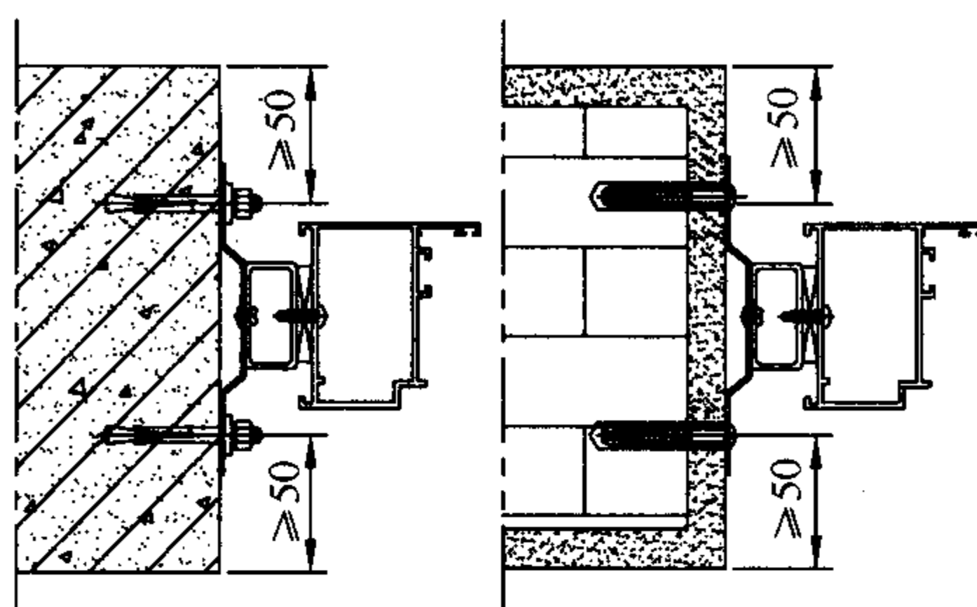
图 7.3.1-1 固定片安装位置
