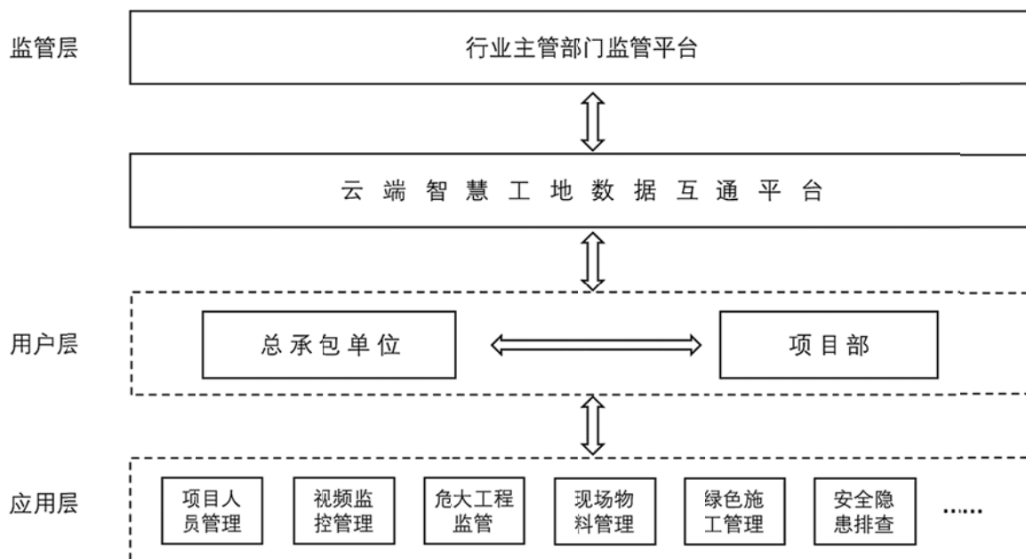
图 3.1 智慧工地管理平台架构图
